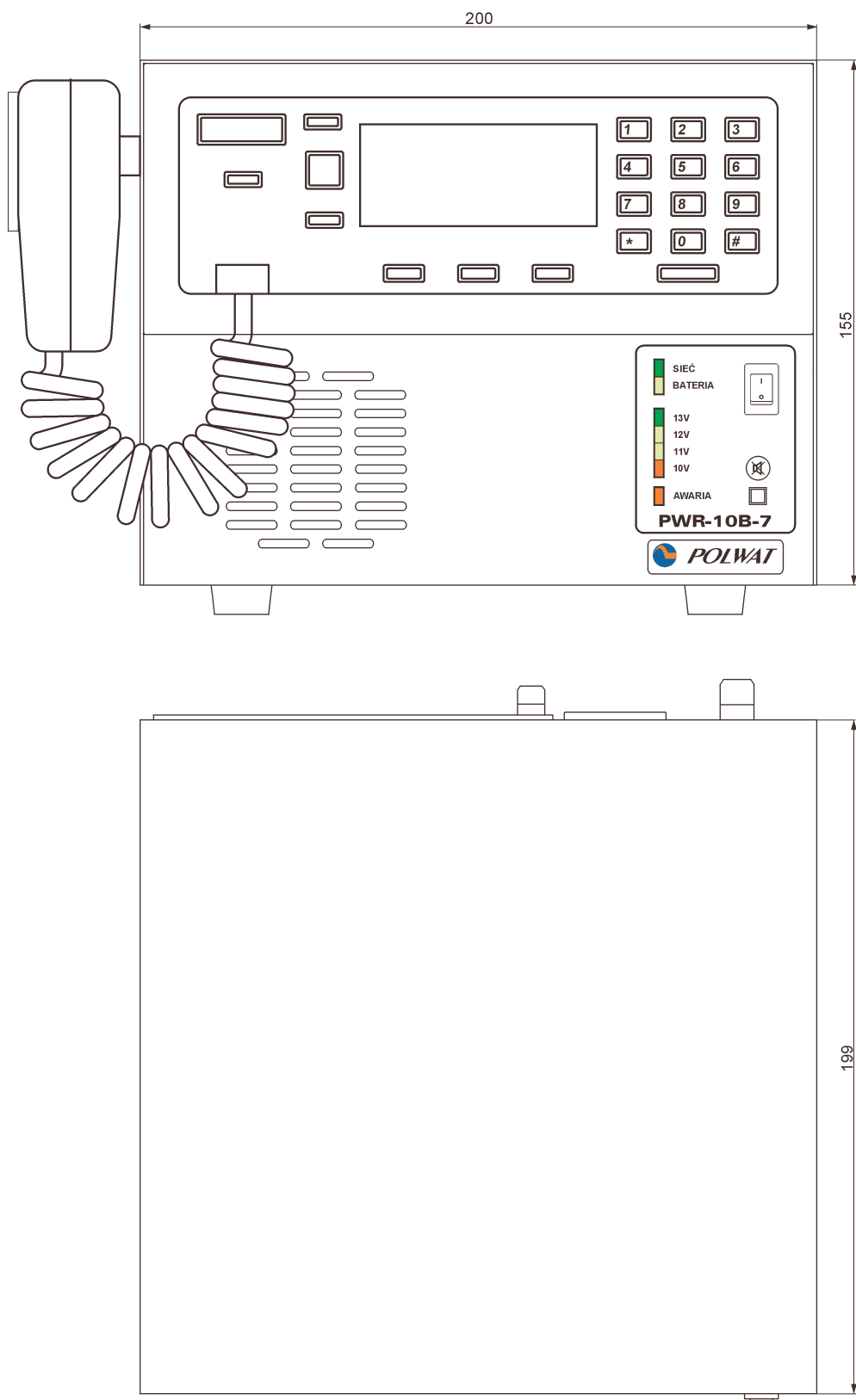
Rys.1. Wymiary gabarytowe zasilacza PWR-10B-7R
